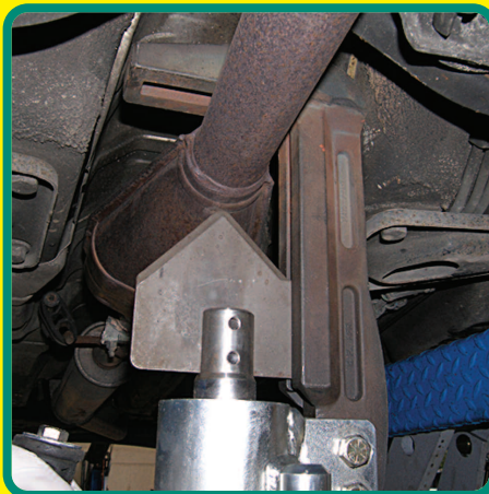
Amenez l'AutoShear au-dessus du conduit d'échappement.
