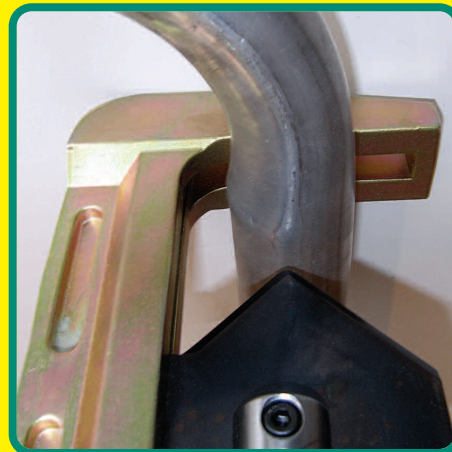
Positionnez le centre de la lame au centre du conduit d'échappement.
